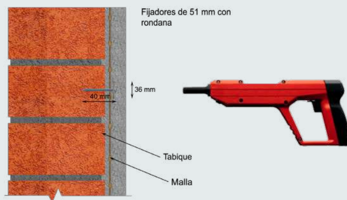
Figura 6.9.13 Anclaje de malla con conectores instalados mediante cargas explosivas de potencia controlada: Fuente: Alcocer (2019).
