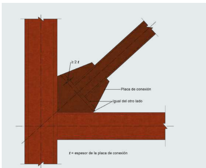
Figura 6.11.16 Requerimientos geométricos para una placa de conexión de contraventeo. Fuente: elaboración propia con base en NTC-Acero (2017).
