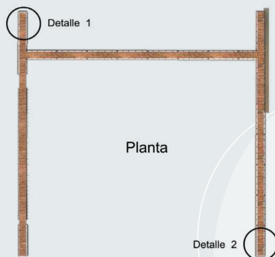
Figura 6.9.14 Colocación de malla de alambre soldado en la superficie de los muros de mampostería. Fuente: elaboración propia con base en NTC-Mampostería (2017).
