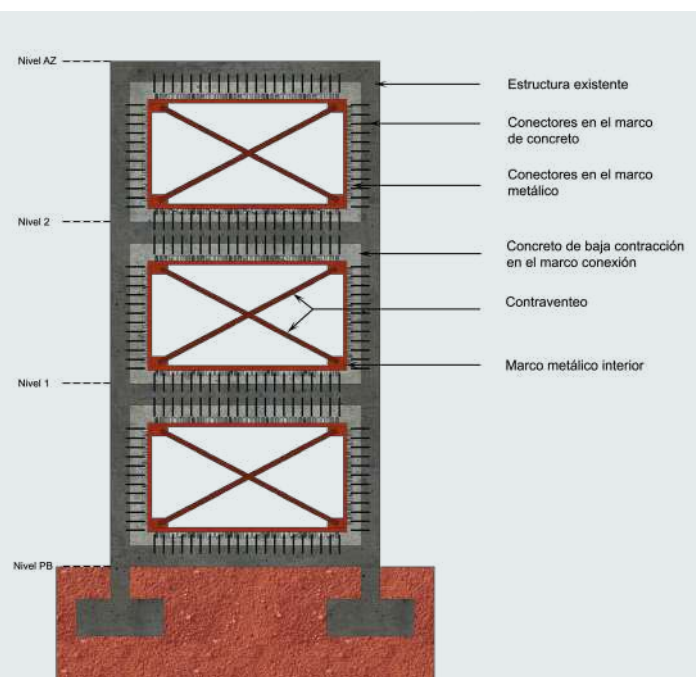
Figura 6.11.9 Contraventeo concéntrico en X dentro de la crujía de un marco de concreto. Fuente: elaboración propia.
