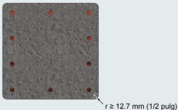
Figura 6.8.3 Esquinas redondeadas en elementos de concreto. Fuente: elaboración propia.
