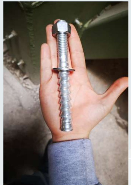
Figura 5.6.1 Tipos de anclas y conectores post-instalados. Fuente: elaboración propia con base en ACI 355.3R, 2011 y archivo personal de Rubén Bautista (2018).
