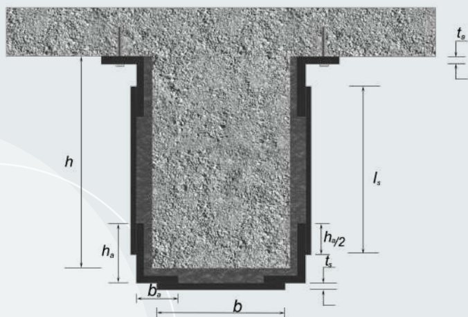
Figura 6.7.10 Sección transversal de viga encamisada con ángulos y solera. Fuente: elaboración propia.
