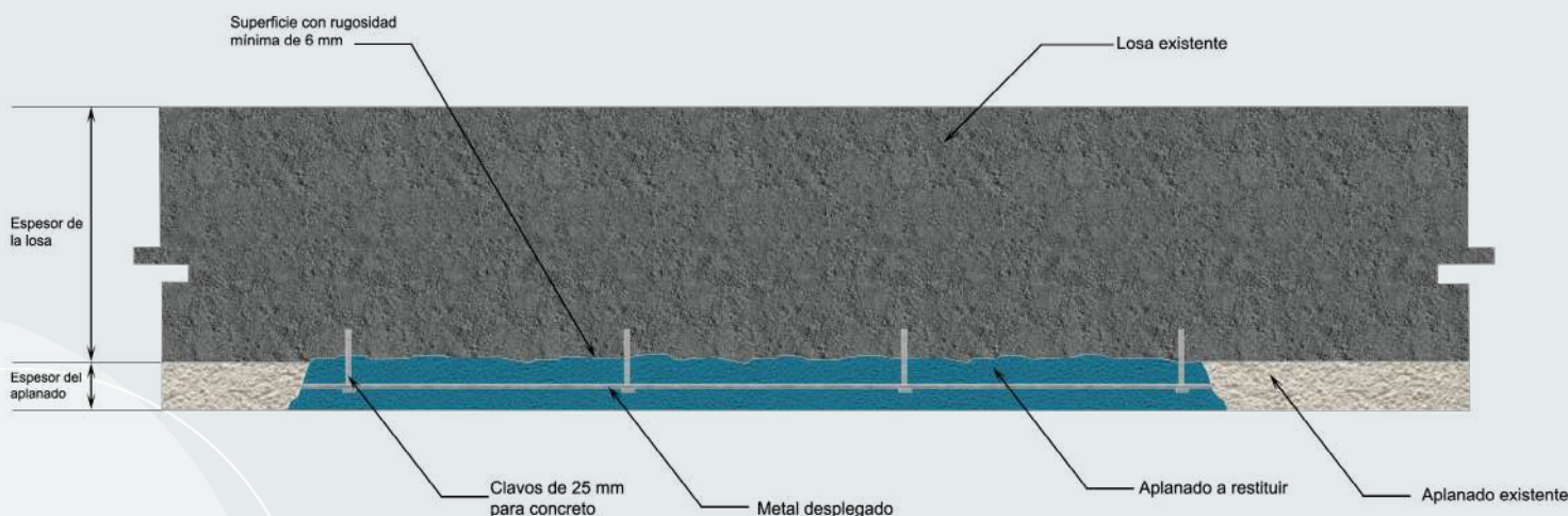
Figura 6.2.4 Restitución de aplanado de losa. Fuente: elaboración propia con base en INIFED (2017b).
