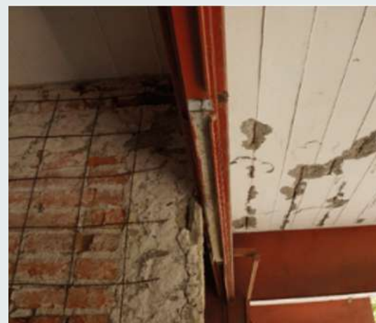
c. Práctica incorrecta de cortar el armado del encamisado en el borde, sin darle continuidad alrededor de él
