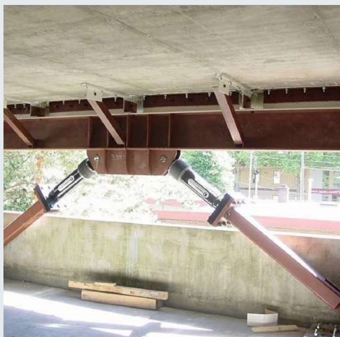
b) Disipadores de energía
