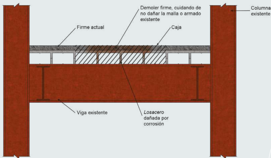
Figura 6.2.3 Reparación de losacero. Fuente: elaboración propia con base en INIFED (2017b).
