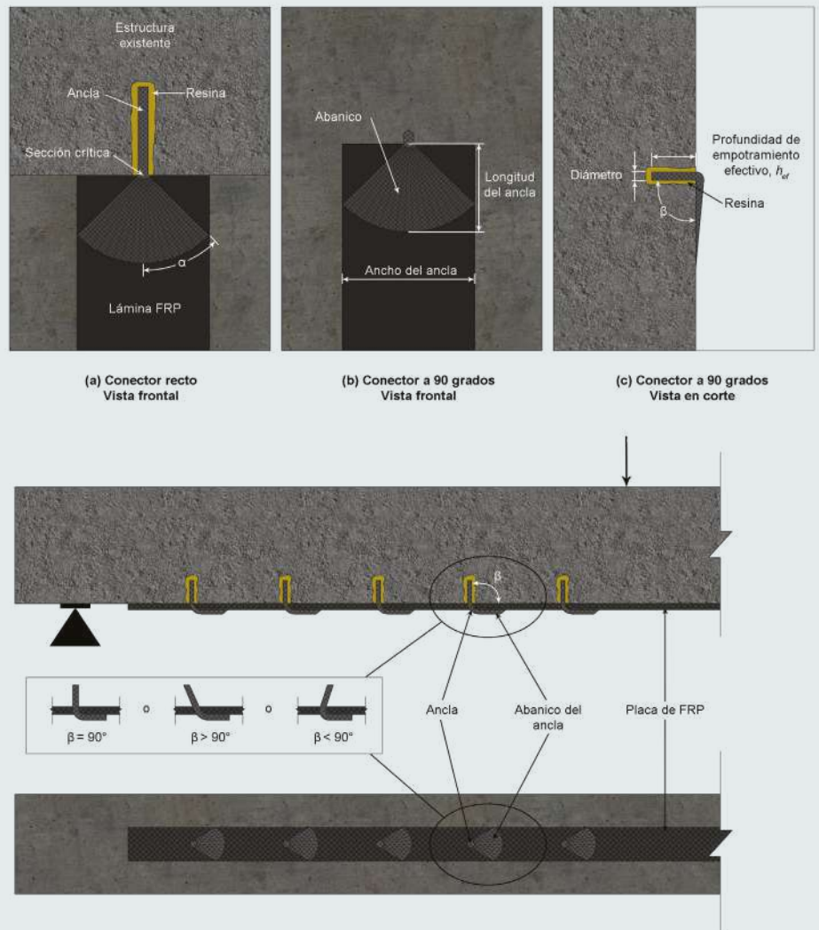
Figura 6.8.9 Tipos de conectores de CPRF. Fuente: elaboración propia con base en Del Rey et al. (2017) y Zhang y Smith (2011).
