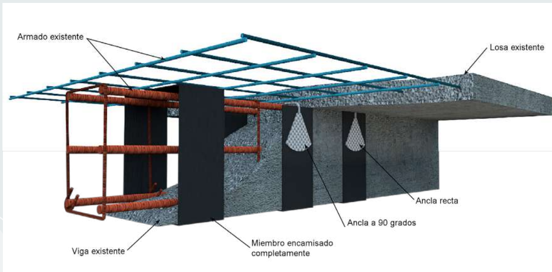
Figura 6.8.11 Ejemplo de uso de conectores de CPRF. Fuente: elaboración propia con base en Del Rey et al. (2017).
