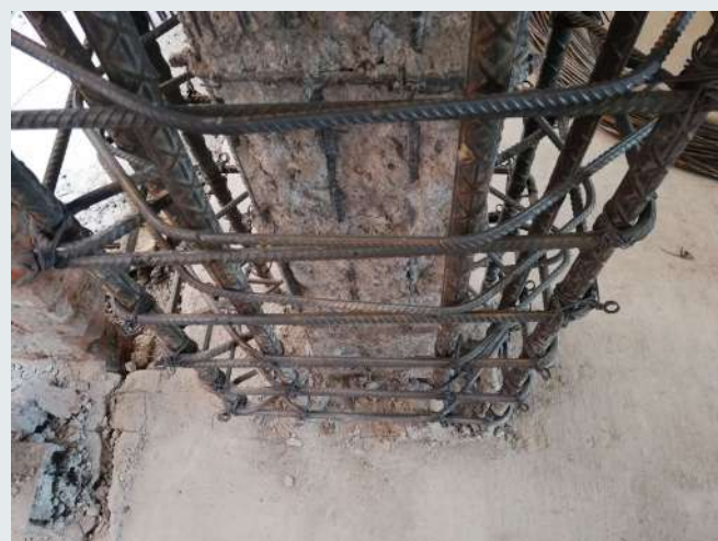
Figura 6.6.13 Práctica incorrecta: estribos con dobleces a 90 grados. Fuente: archivo personal de Víctor Cruz (2019).
