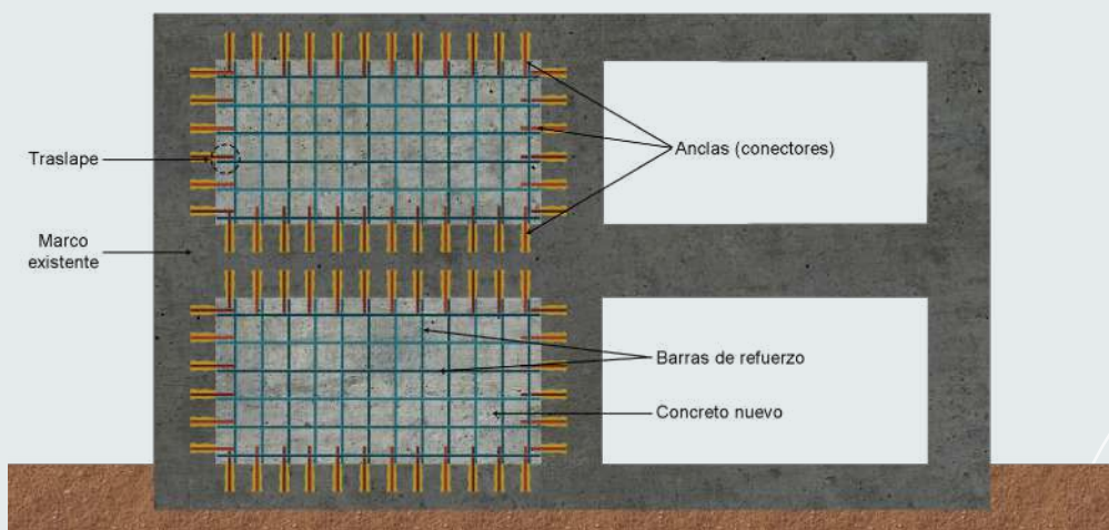
Figura 6.5.10 Anclas para unir elementos de concreto. Fuente: elaboración propia con base en Terán (2009).
