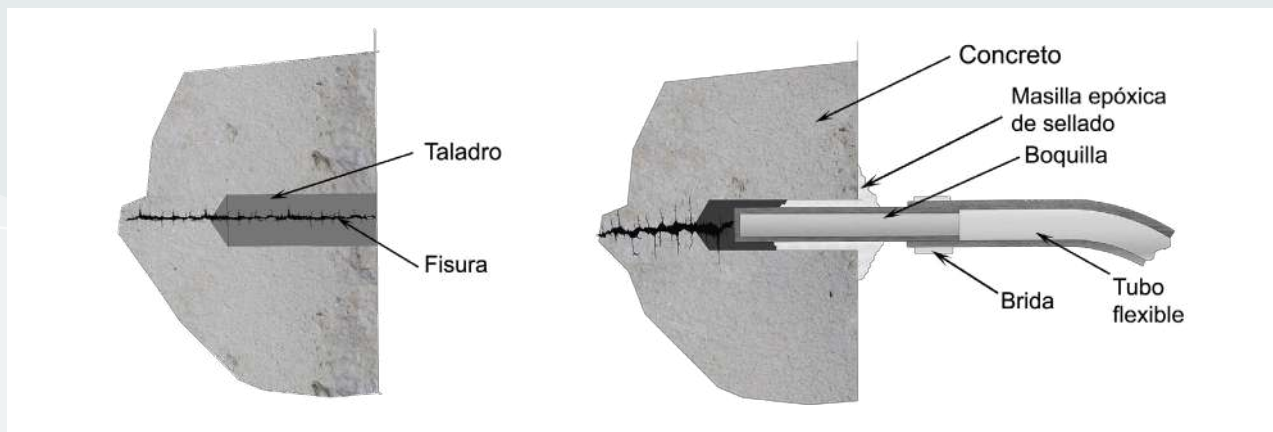
Figura 6.3.2 Diagrama de perforación de la grieta. Fuente: elaboración propia con base en Fernández (1981).
