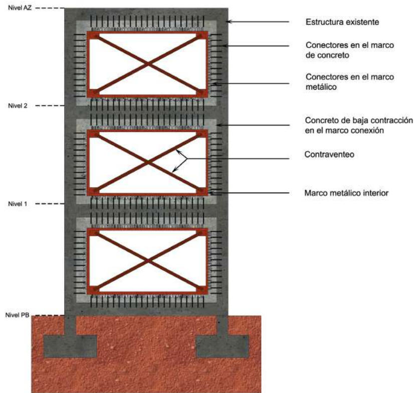
Figura 6.11.20 Elevación de contraventeos conectados a la estructura existente mediante marcos metálicos perimetrales y marcos de concreto de baja contracción. Fuente: elaboración propia.
