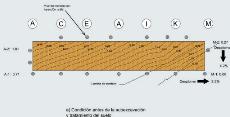
Figura 6.16.13 Aplicación de los pilares de mortero para recimentar y renivelar un edificio. Fuente: elaboración propia con base en Santoyo y Miranda (1997).
