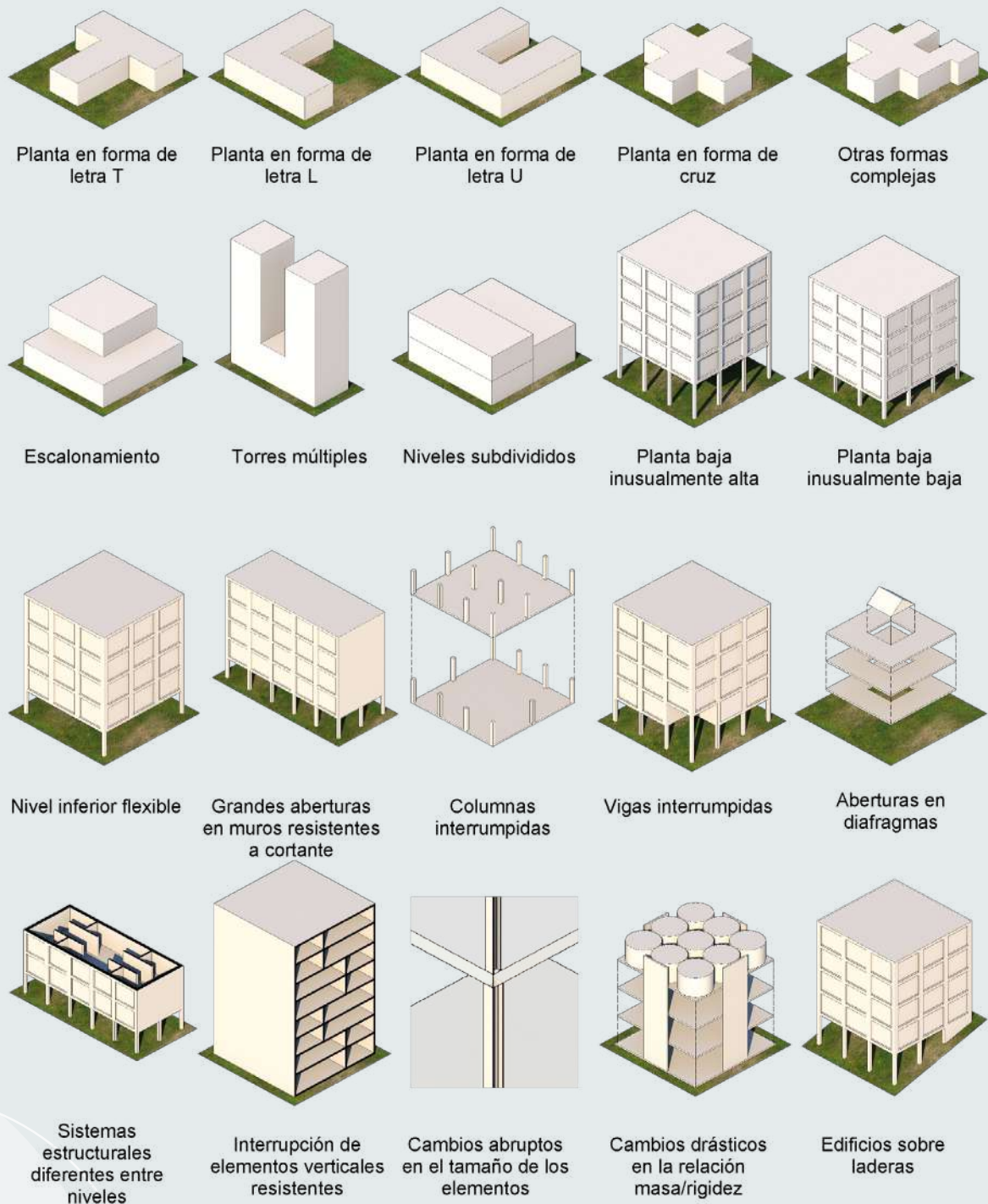
Figura 2.6.1 Estructuras irregulares. Fuente: elaboración propia con base en Arnold y Reitherman (1991).
