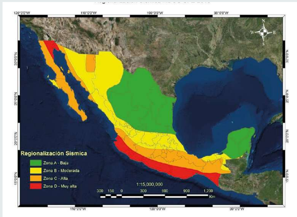
Figura 1.1.1 Regionalización sísmica de México. Fuente: Comisión Federal de Electricidad (2017b).
