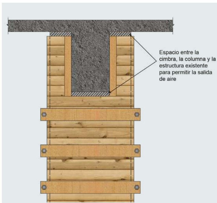
Figura 6.6.18 Ejemplo de cimbra de columna encamisada diseñada para facilitar la salida de aire del concreto. Fuente: elaboración propia.
