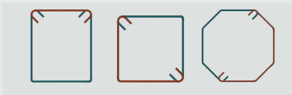
Figura 6.6.12 Estribos de dos piezas aceptables para encamisado de concreto. Fuente: elaboración propia.
