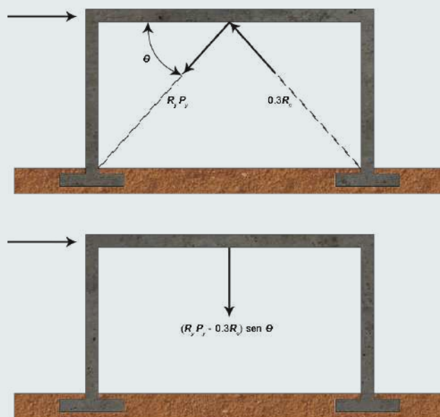
Figura 6.11.14 Distribución de fuerzas máximas en marcos con contraventeos en V invertida. Fuente: elaboración propia.
