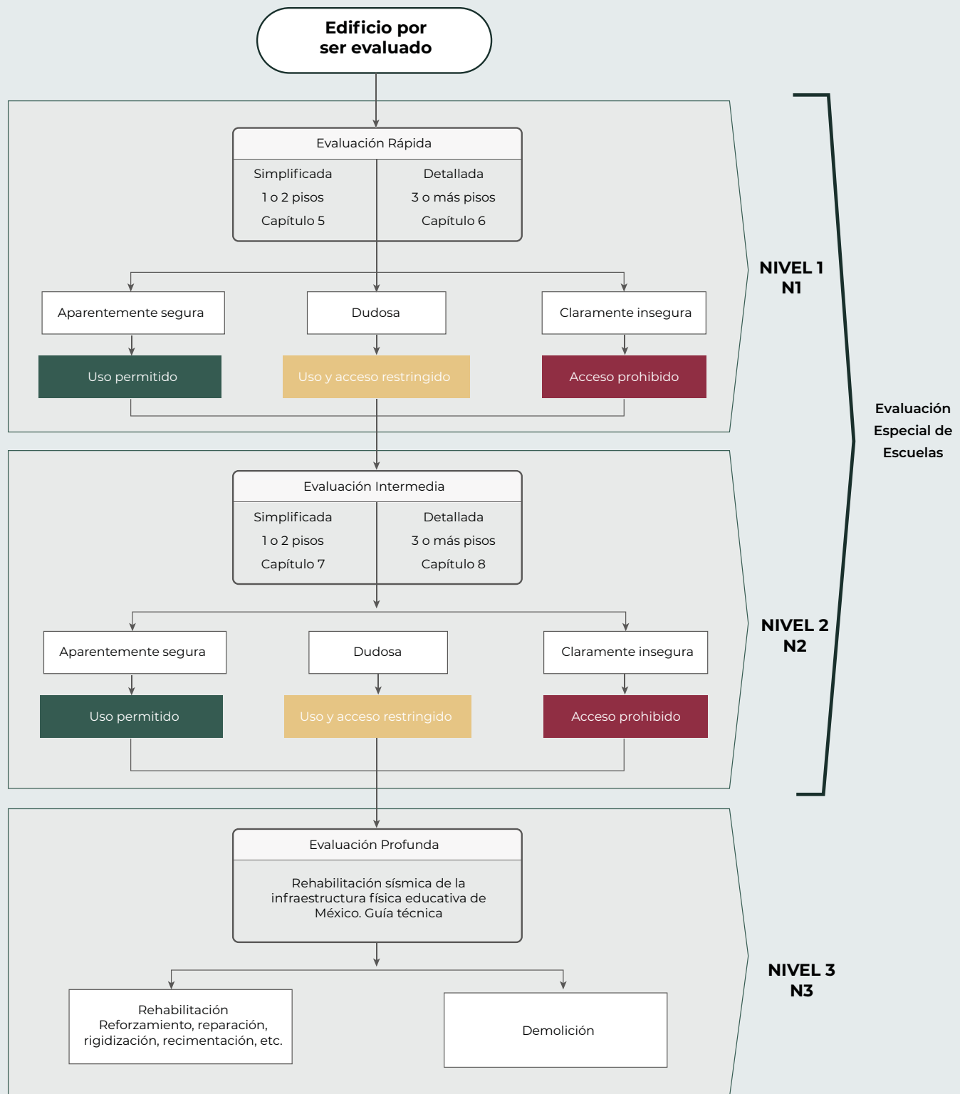
Figura 1.3.1 Diagrama de flujo del procedimiento de evaluación postsísmica de un edificio escolar. Fuente: elaboración propia (2020).
