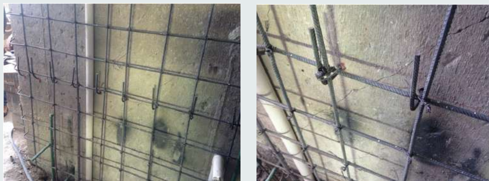
Figura 6.10.6 Incremento de espesor de muros existentes y detalle de anclas a 90 grados. Fuente: archivo personal de Bernardo Moctezuma (2019).
