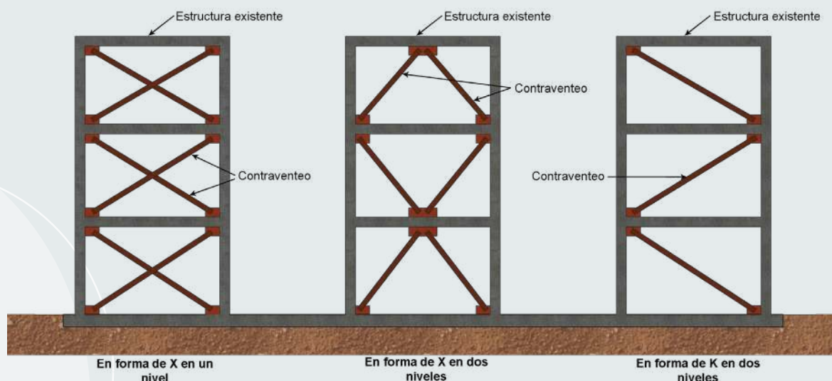
Figura 6.11.1 Contraventeos en X y K permitidos para la rehabilitación de estructuras. Fuente: elaboración propia.
