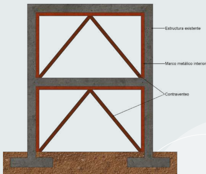
Figura 6.11.15 Marco metálico conectado a un marco de concreto cuando se usan contraventeos concéntricos tipo V invertida. Fuente: elaboración propia.
