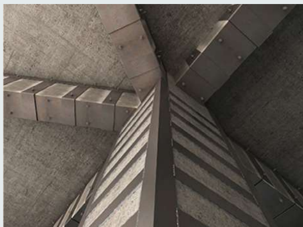
Figura 6.7.7 Ejemplo de encamisado con armadura de ángulos y soleras, con y sin conectores. Fuente: Horse Construction Company China, www.horseseen.com
