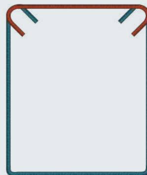
Figura 6.6.11 Estribo de dos piezas aceptable para encamisado de vigas de concreto. Fuente: elaboración propia.
